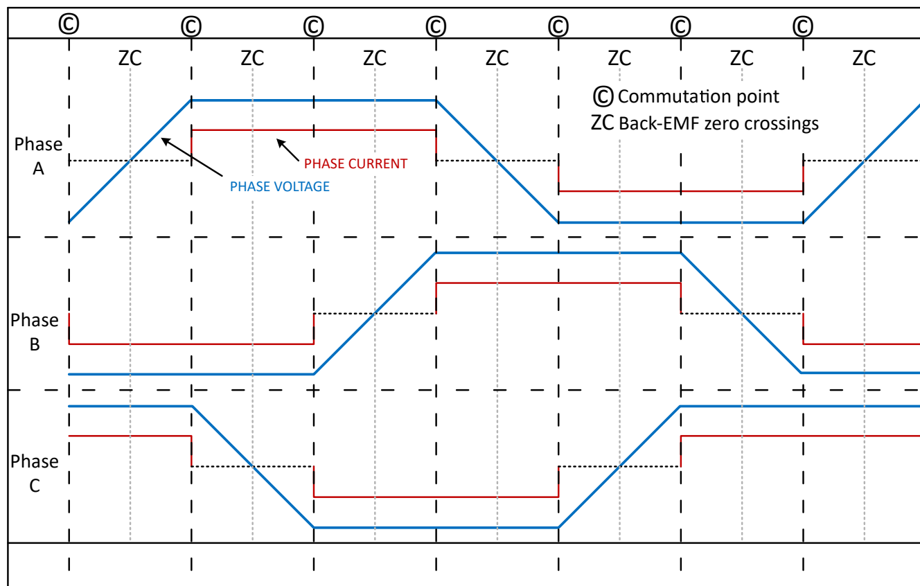
图 7-27. 120° commutation
