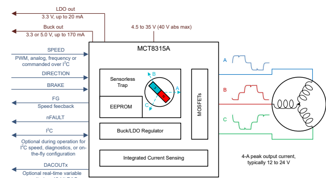
简化原理图
