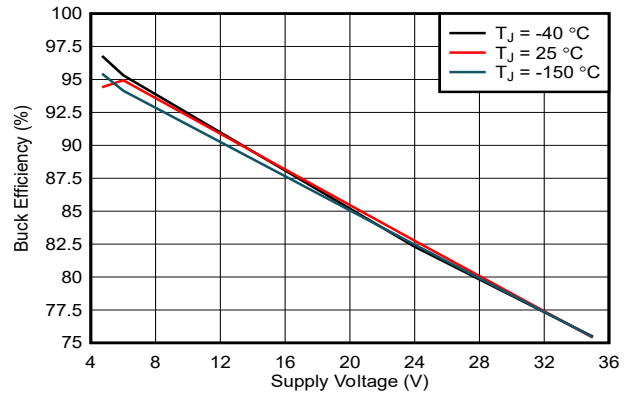
图 5-2. 降压稳压器在电源电压下的效率
