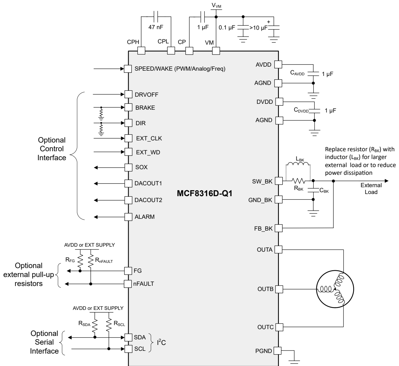
图 9-1. 示例应用原理图
