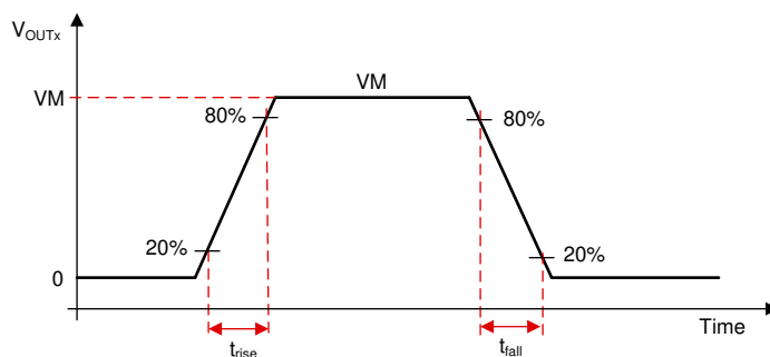
图 6-10. 压摆率时序
