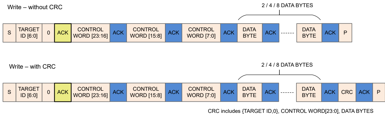
图 6-65. I 2 C 写入事务序列
