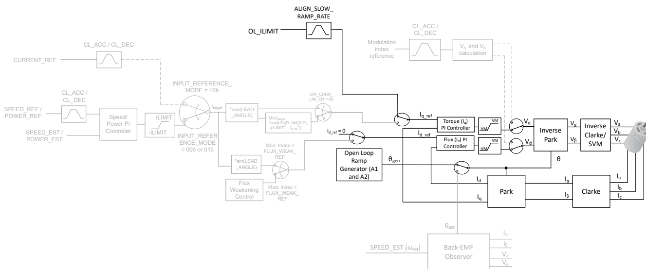
图 6-35. 开环
