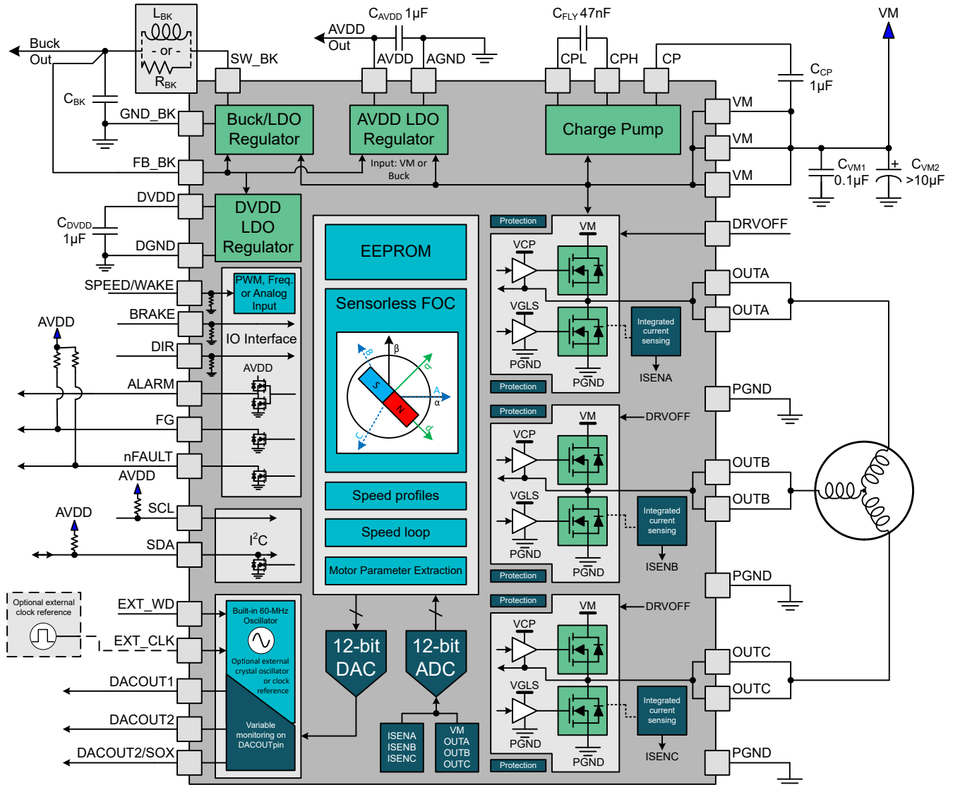
图 6-1. MCF8316D-Q1 功能方框图
