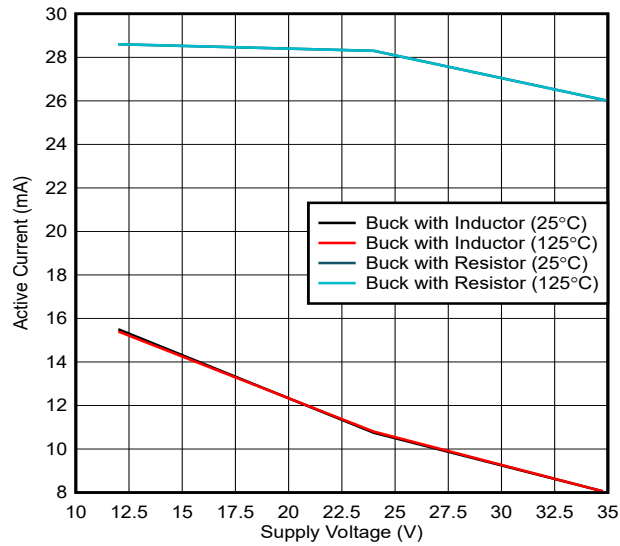
图 5-1. 电源电流与电源电压间的关系
