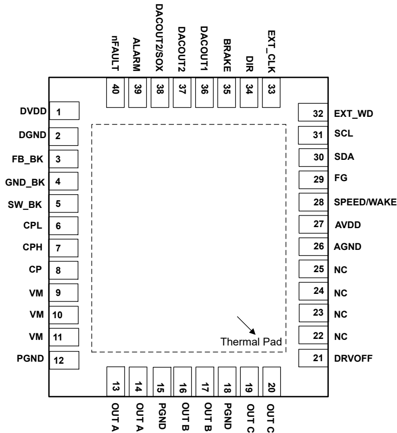
图 4-1. MCF8316D-Q1，40 引脚 VQFN（带有外露散热焊盘），顶视图
