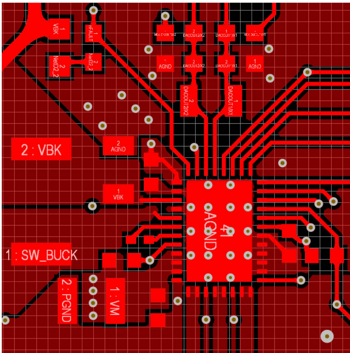
图 9-12. 推荐布局示例
