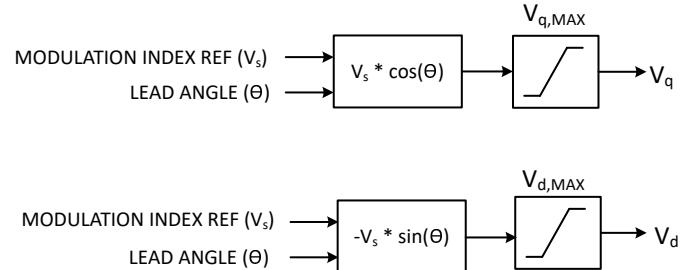
图 6-44. 开环电压控制
