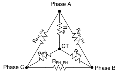
图 6-46. 电机电阻
