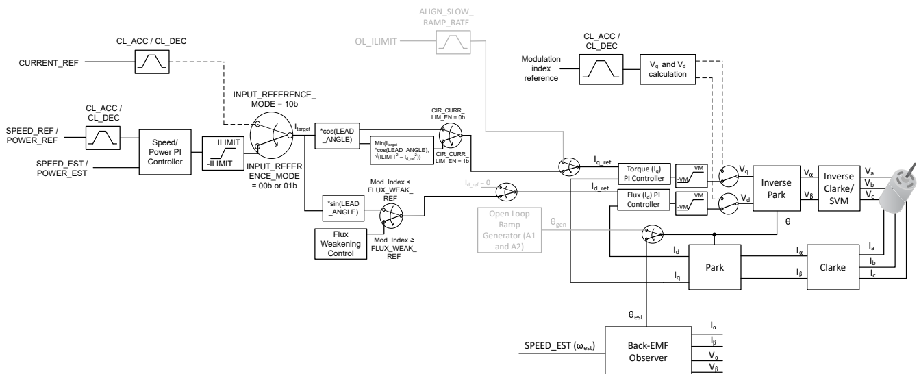
图 6-37. 开闭环转换控制方框图
