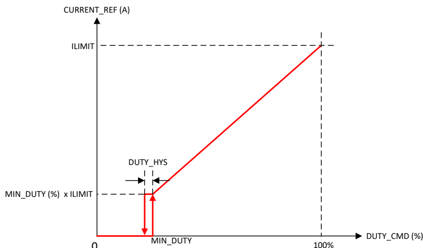
图 6-26. 电流基准传递函数
