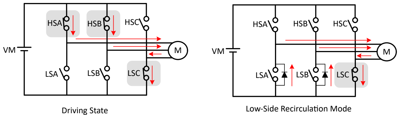
图 6-54. 低侧再循环
