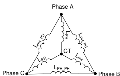
图 6-47. 电机电感
