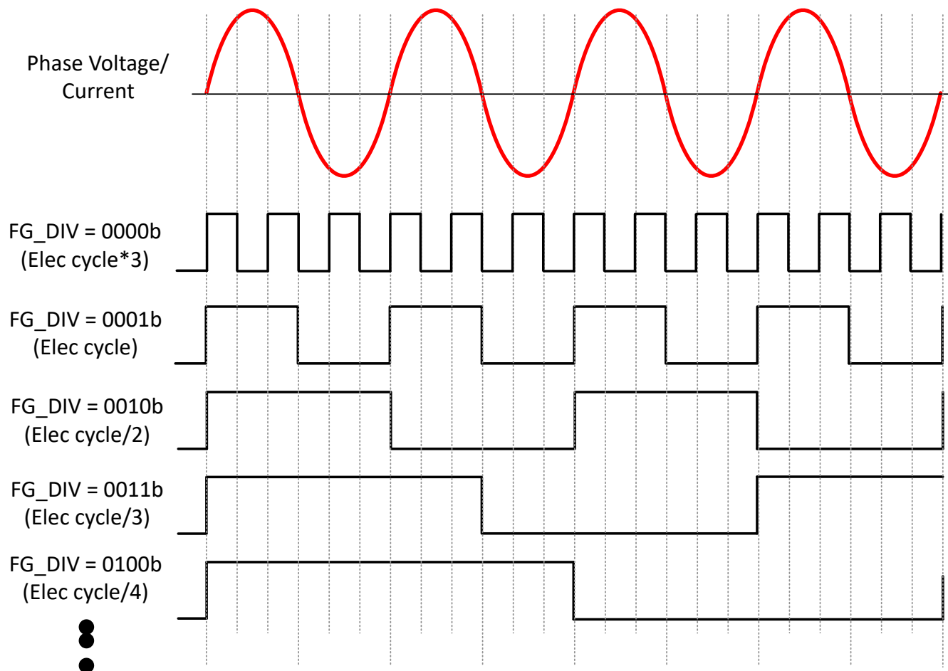
图 6-58. FG 分频器
