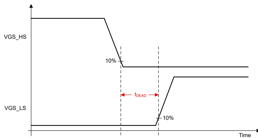
图 6-12. 死区时间
