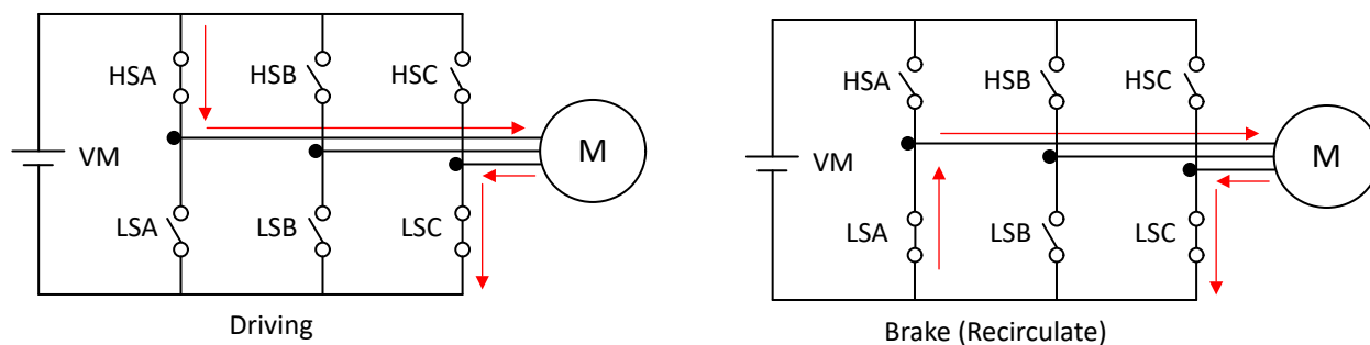
图 6-32. IPD 释放模式 - 制动 (0b)
