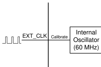
图 6-64. 外部时钟基准
