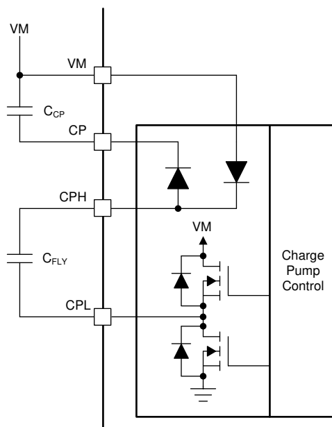
图 6-8. 电荷泵
