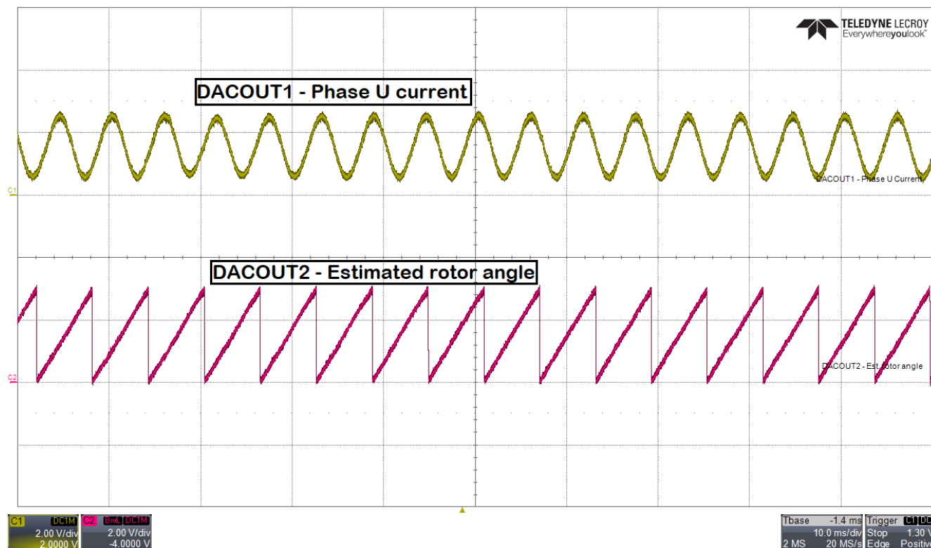
图 9-10. DACOUT1 和 DACOUT2
