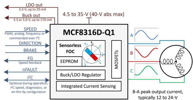
图 3-1. 简化版原理图
