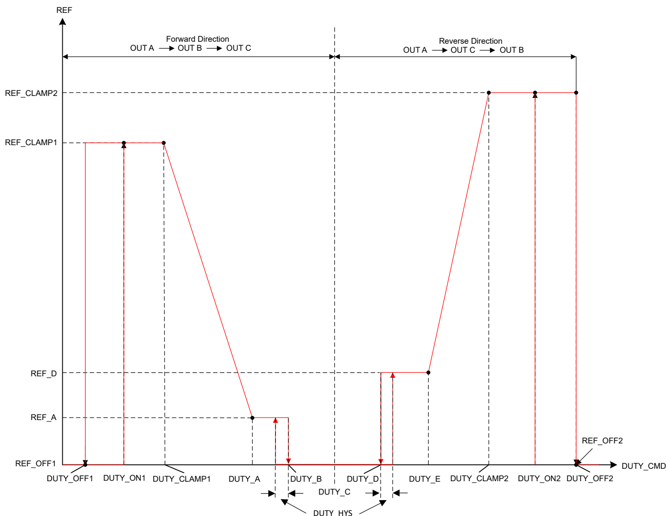
图 7-20. 正向反向控制曲线
