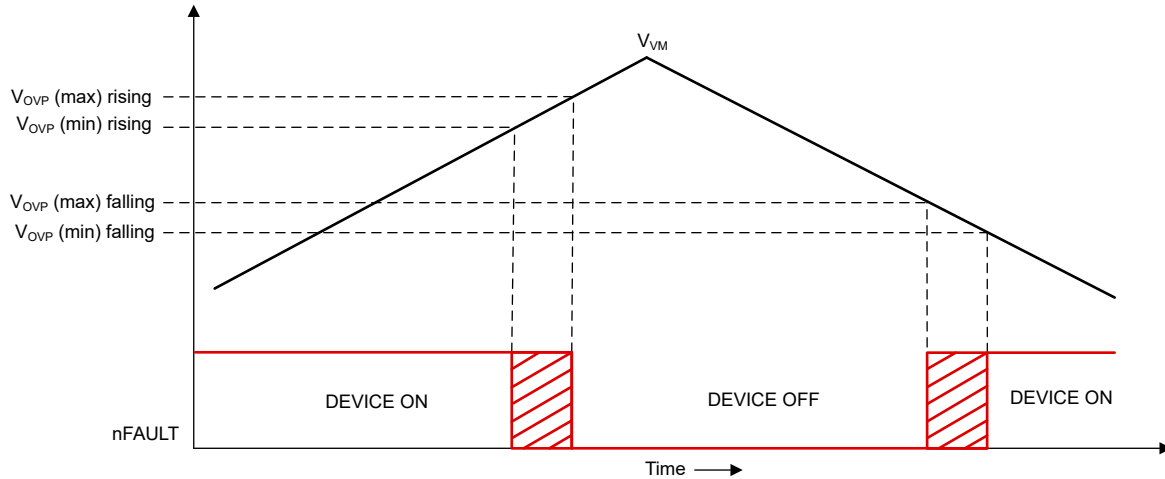
图 7-61. 过压保护
