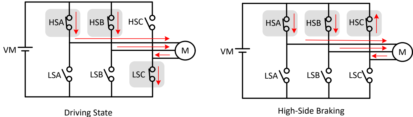
图 7-57. 高侧制动
