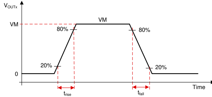
图 7-10. 压摆率时序
