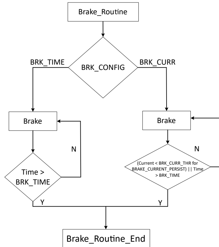
图 7-23. Brake Routine
