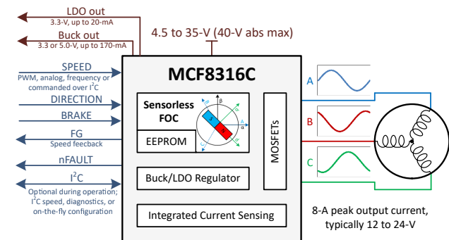
简化原理图
