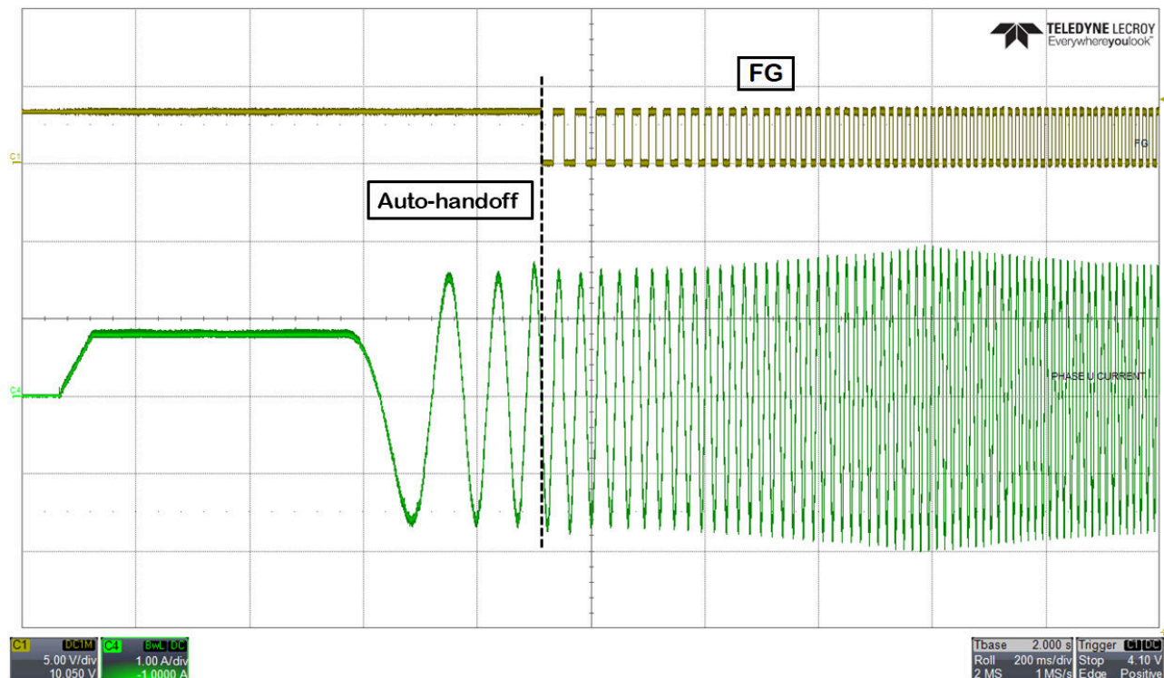
图 8-7. Auto-handoff
