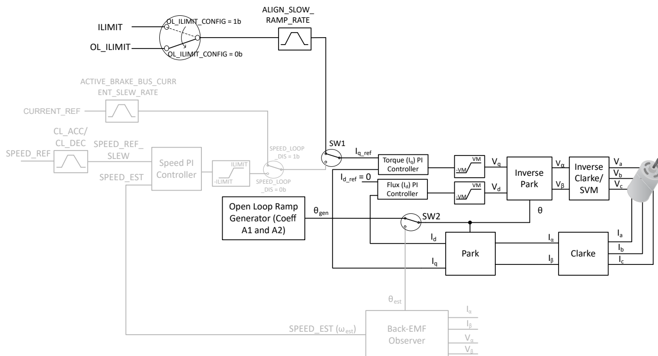
图 7-29. Open Loop
