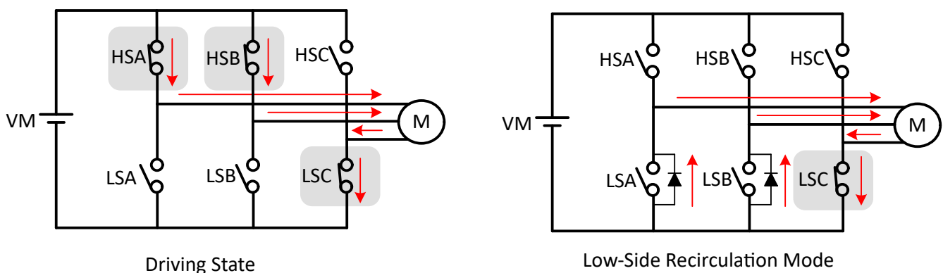
图 6-56. 低侧再循环
