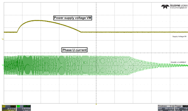
图 9-8. 禁用 AVS 时的电源电压和相电流波形
