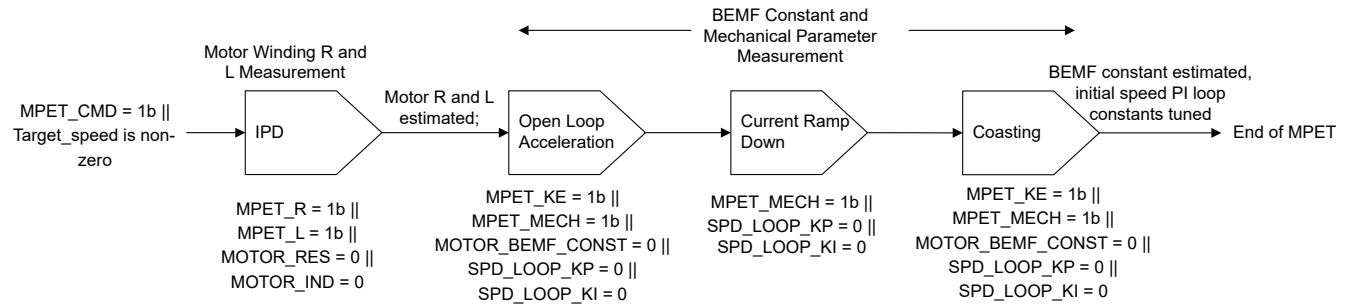
图 6-42. MPET 序列
