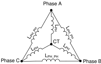
图 6-40. 电机电感
