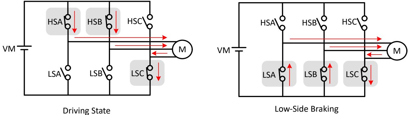
图 6-46. 低侧制动
