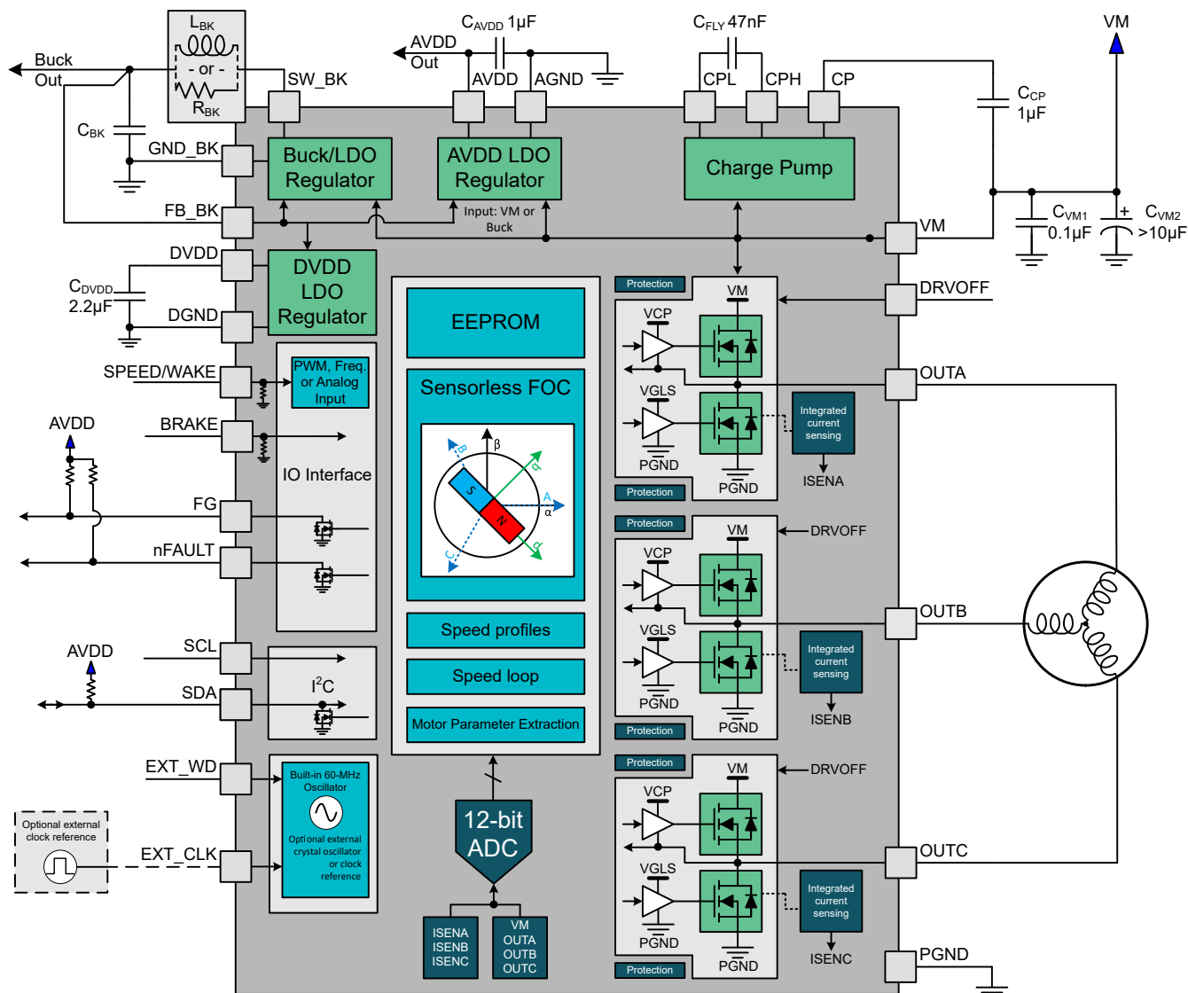
图 6-3. MCF8315C-Q1 (PWP) 功能方框图
