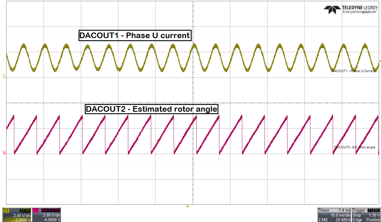
图 9-10. DACOUT1 和 DACOUT2
