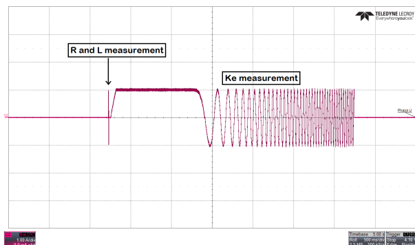
图 9-3. MPET - 相电流
