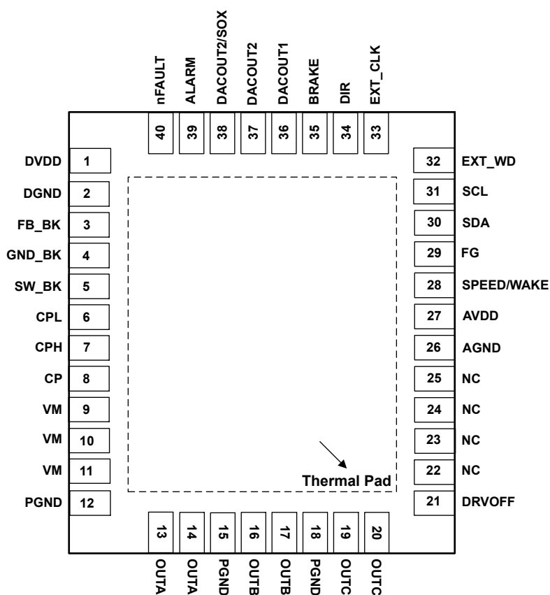
图 4-1. MCF8315C-Q1，40 引脚 VQFN（带有外露散热焊盘），顶视图
