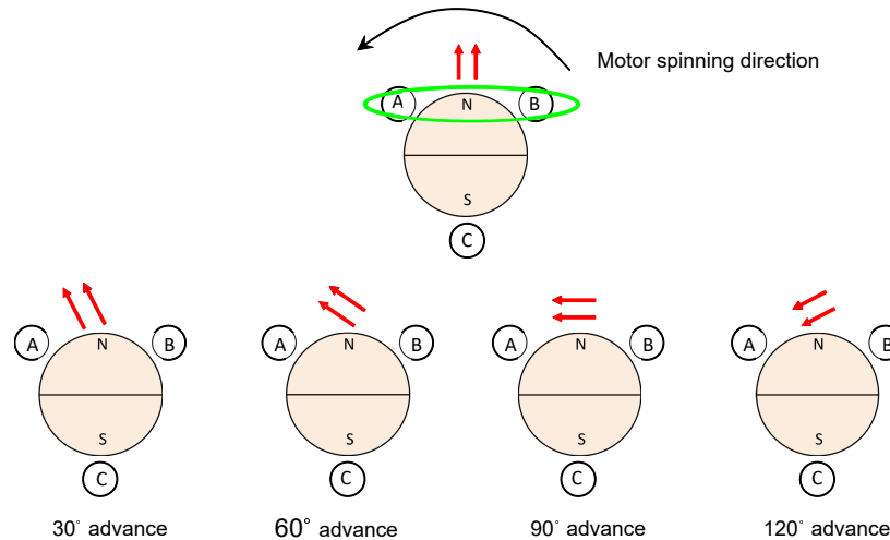
图 6-30. IPD 超前角度
