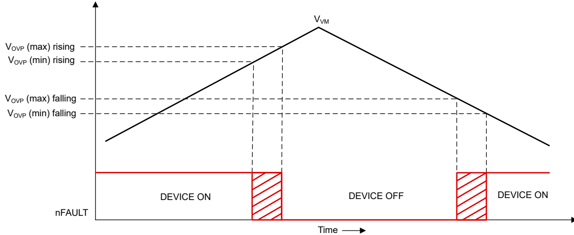
图 6-51. 过压保护
