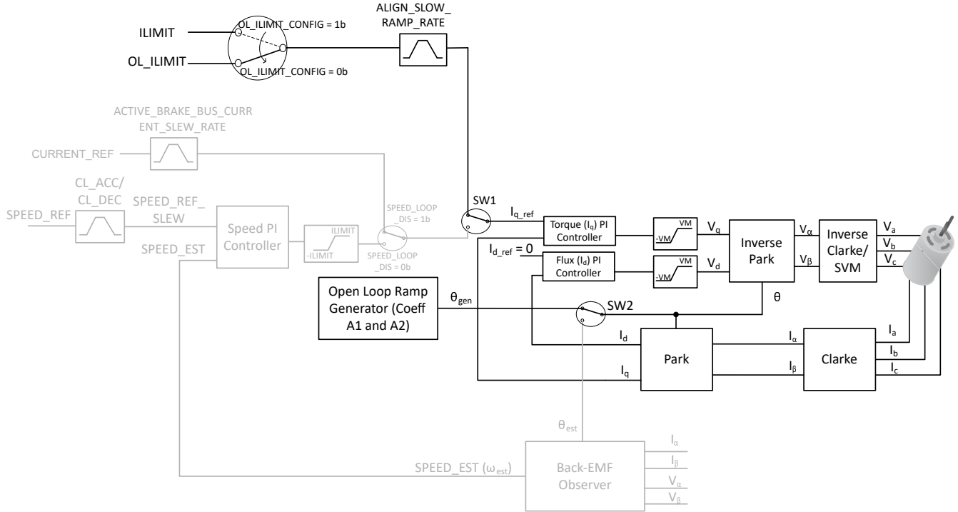
图 6-30. 开环
