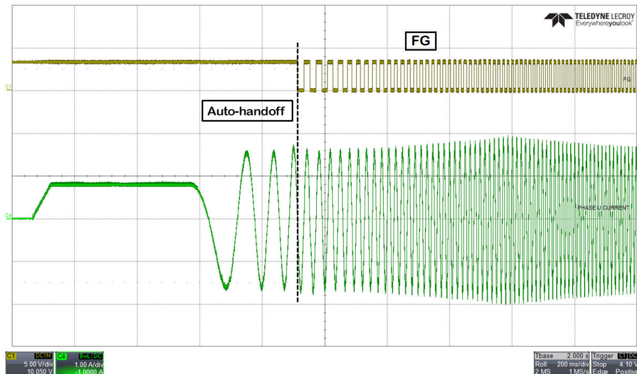
图 7-7. 自动转换
