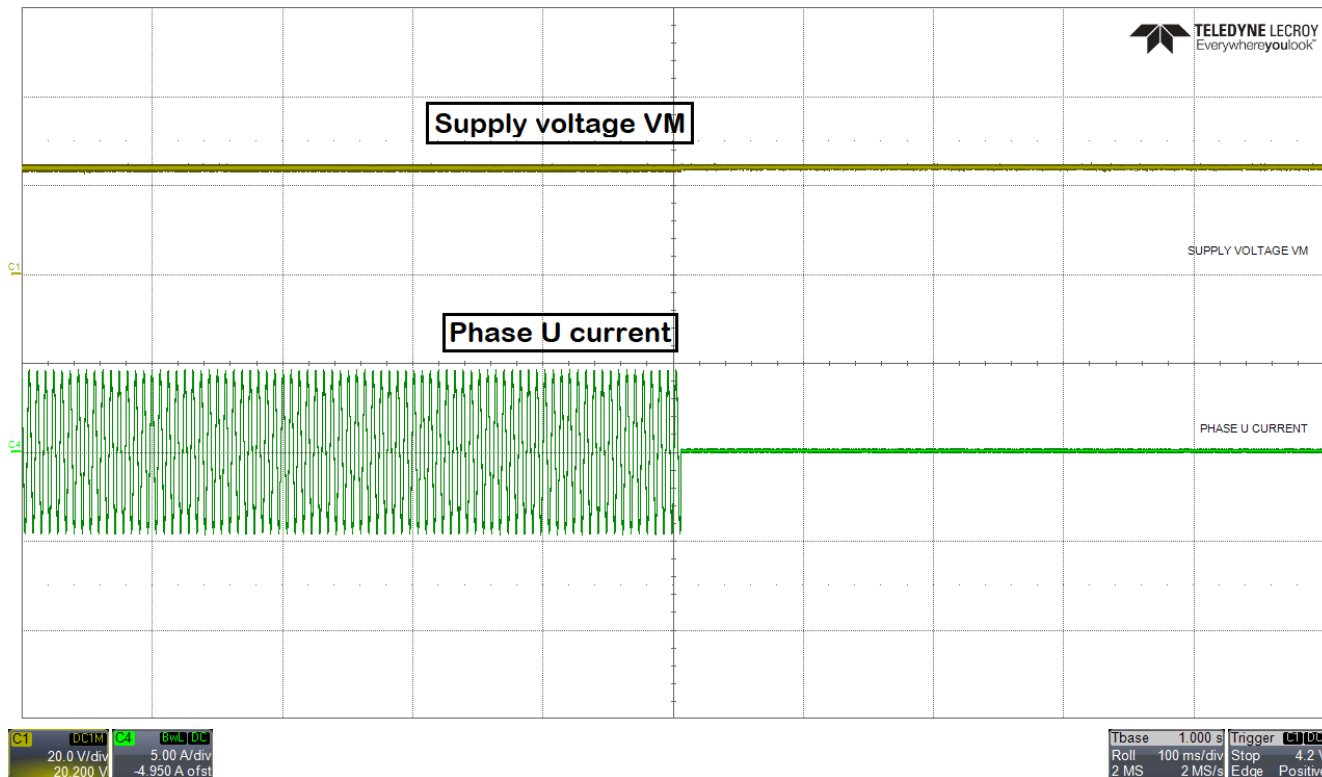
图 8-9. Motor stop - recirculation mode
