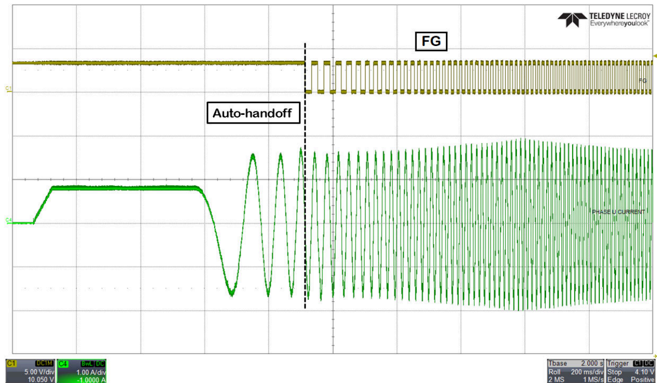
图 8-8. Auto-handoff
