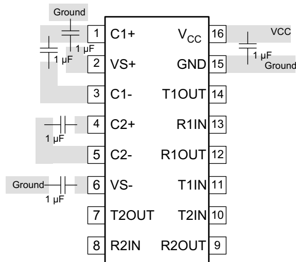
图 8-4. Layout Schematic
