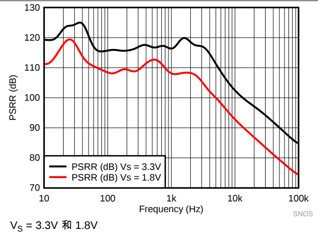
图 22. PSRR 与频率间的关系
