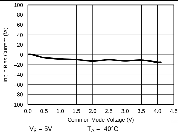
图 16. 输入偏置电流与共模电压间的关系
