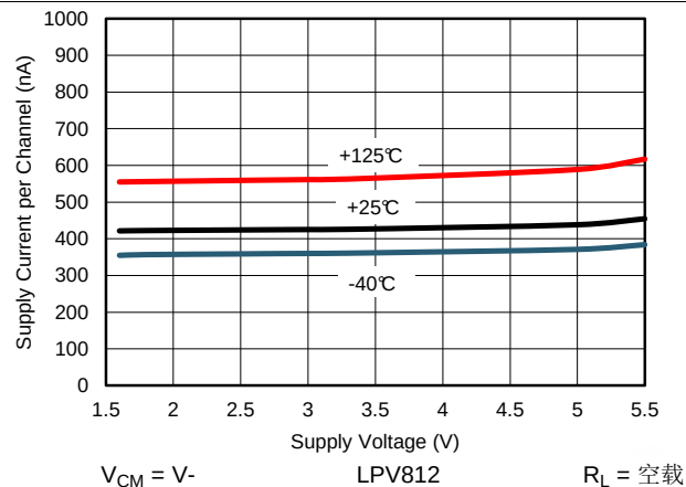
图 10. 电源电流与电源电压间的关系, LPV812
