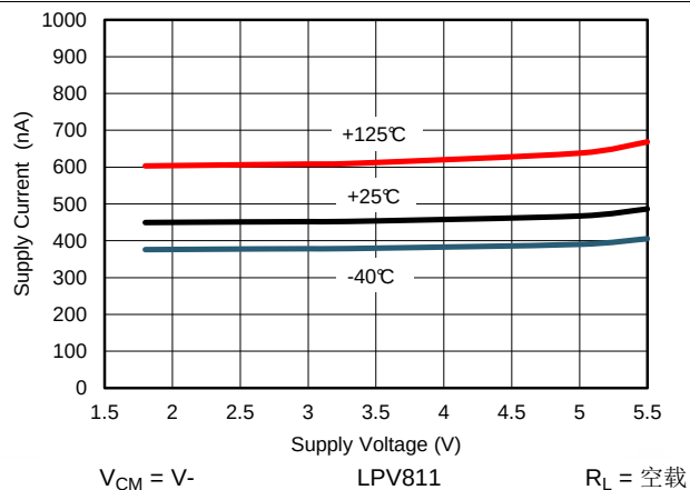
图 9. 电源电流与电源电压间的关系, LPV811
