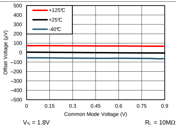
图 11. 典型偏移电压与共模电压间的关系
