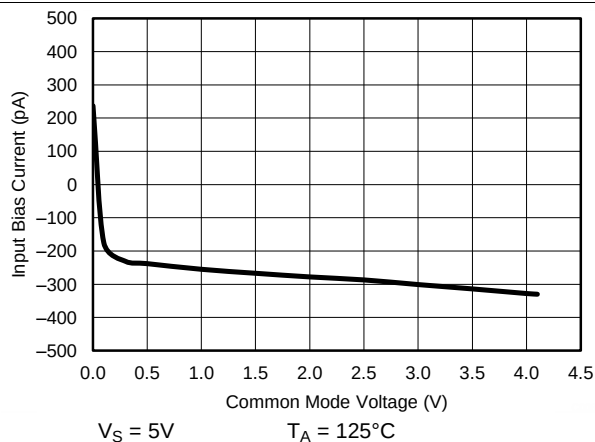
图 20. 输入偏置电流与共模电压间的关系
