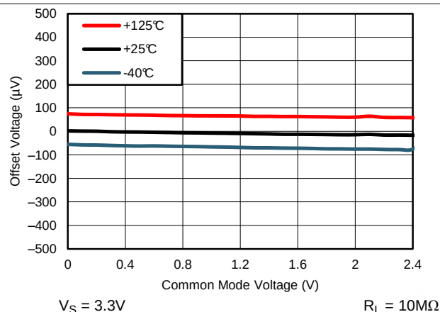
图 12. 典型偏移电压与共模电压间的关系
