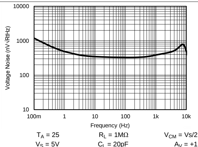
图 42. 输入电压噪声与频率间的关系
