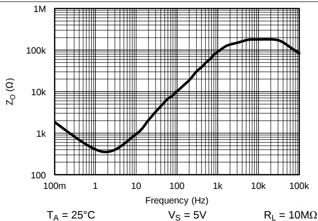
图 40. 开环输出阻抗
