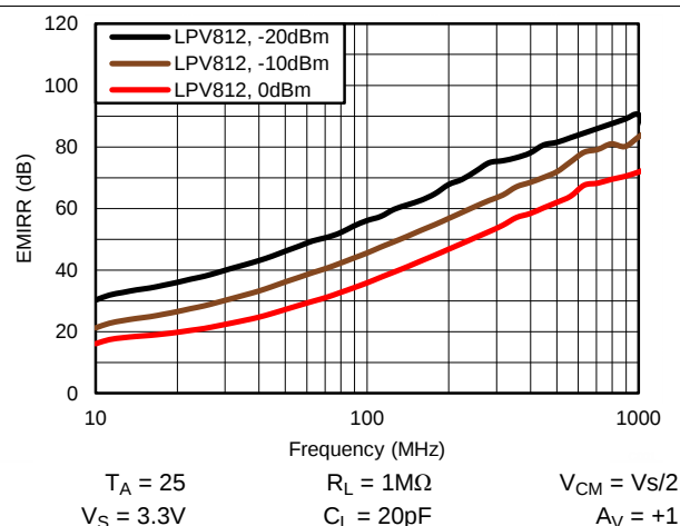
图 44. EMIRR 性能
