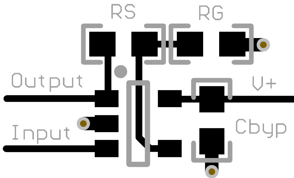
图 7-9. Noninverting Layout Example
