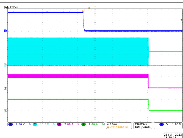
图 8-7. 在 ADIM = 100%、500Hz 时关断
