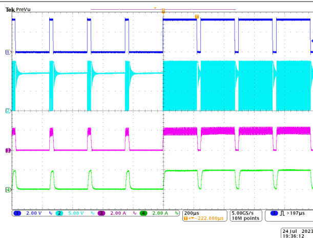
图 8-16. ADIM = 100%、1kHz 且 F_{SW} = 400\text{kHz} 时的 LED 电流纹波
