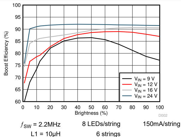
图 5-3. Boost Efficiency
