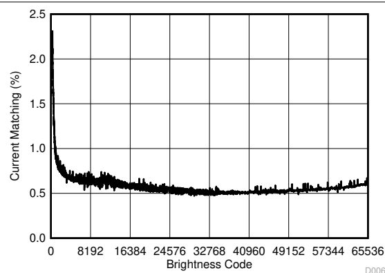
图 5-7. Current Matching
