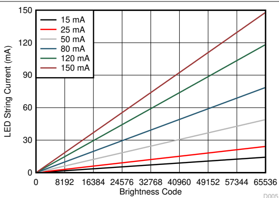
图 5-6. Current Linearity
