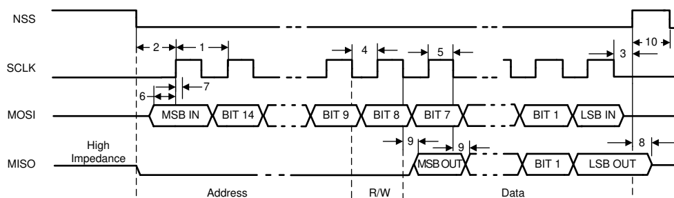
图 5-2. SPI Timing Diagram
