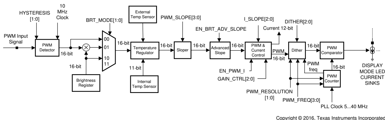
图 6-9. PWM Data Flow Calculation
