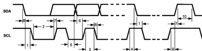
图 5-1. I 2 C Timing
