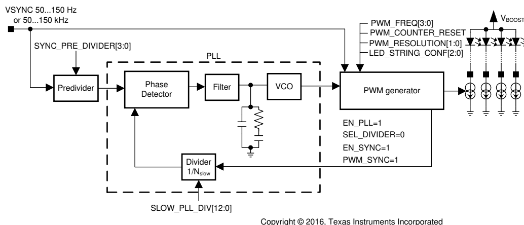
图 6-4. PWM Synchronization With External VSYNC Input
