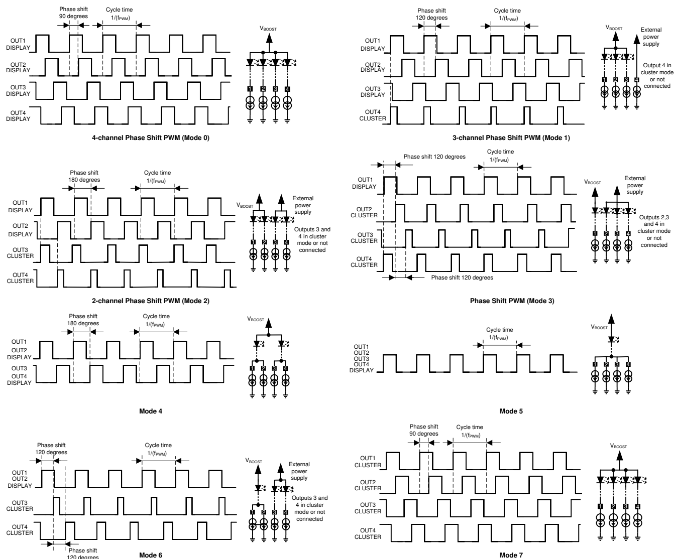
图 6-10. Phase Shift Modes
