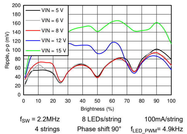
图 5-8. Boost Ripple
