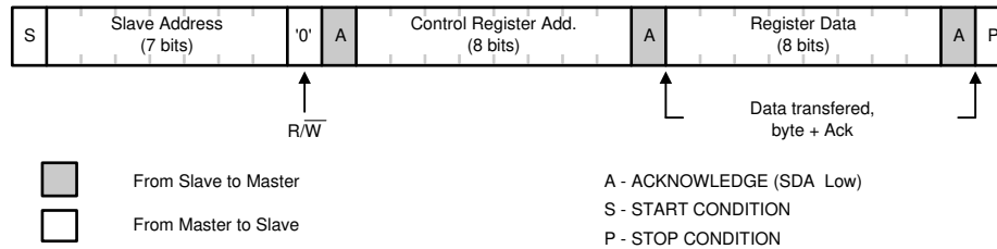
图 6-43. Register Write Format
