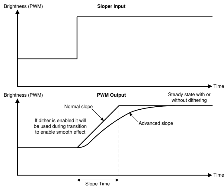
图 6-6. Sloper Operation
