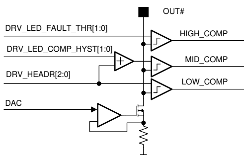
图 6-20. Output Voltage Comparators
