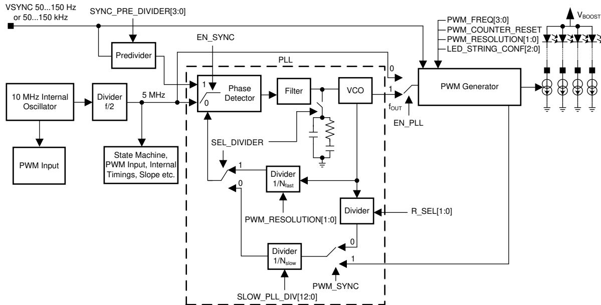
图 6-1. PLL Clock Generation
