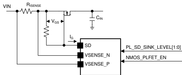
图 6-18. Power-line FET Control
