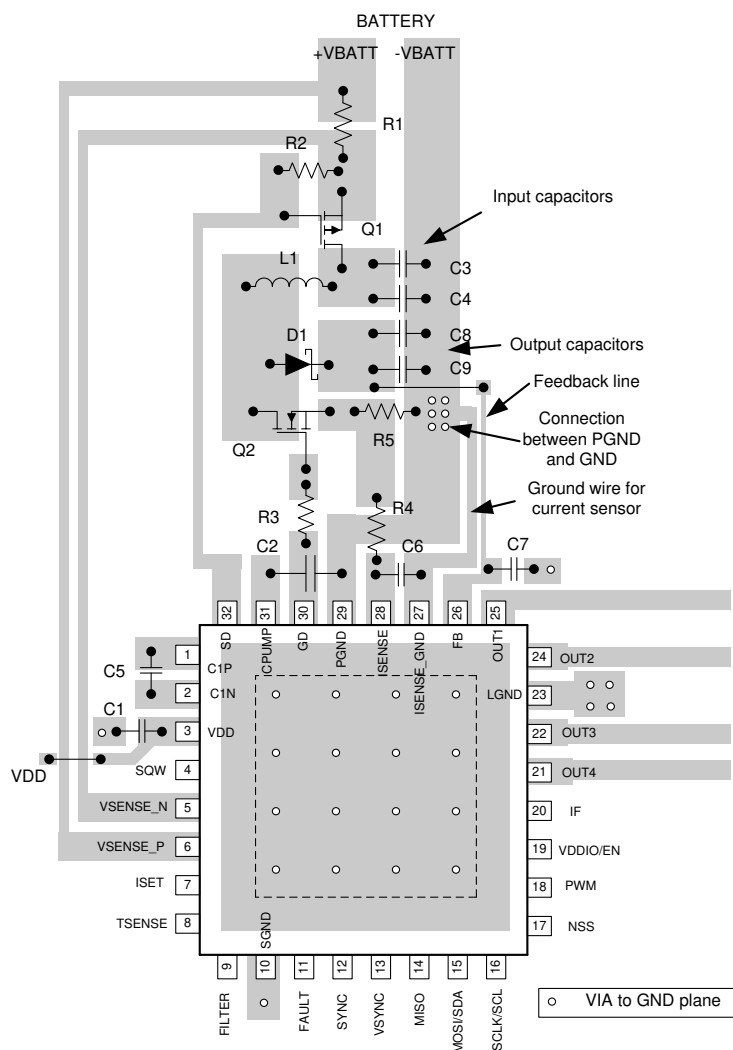
图 7-15. LP8860-Q1 Layout
