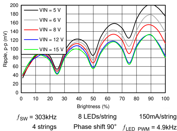
图 5-7. Boost Ripple
