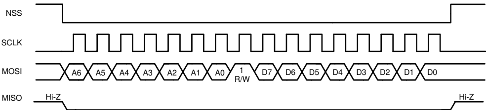
图 6-37. SPI Write Cycle
