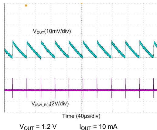
图 9-14. Buck Output Voltage Ripple, PFM Mode
