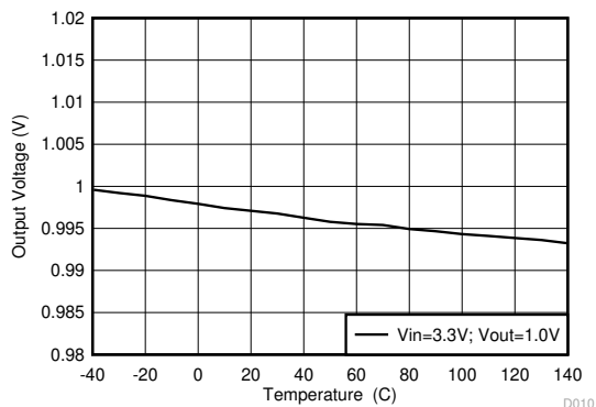
图 8-9. Buck Output Voltage vs Temperature
