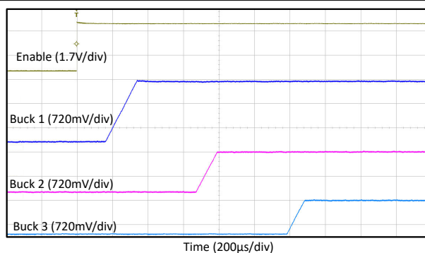
图 6-4. Startup, LP876242B0
