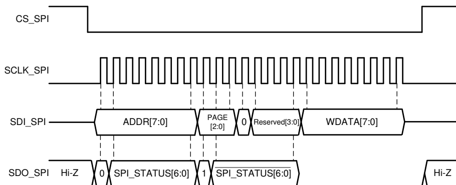
图 7-56. SPI Write Cycle
