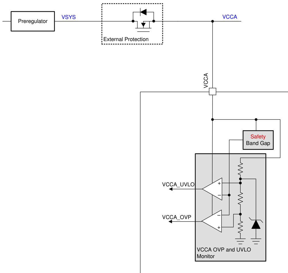
图 7-2. VCCA Monitor
