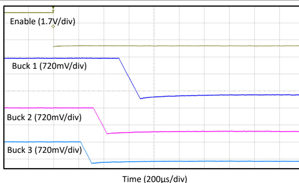
图 6-5. Shutdown, LP876242B0
