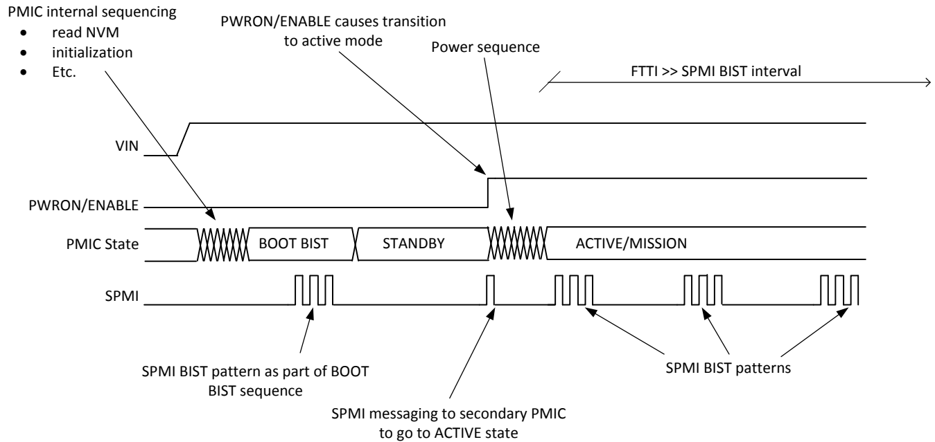
图 7-45. SPMI-BIST Operation
