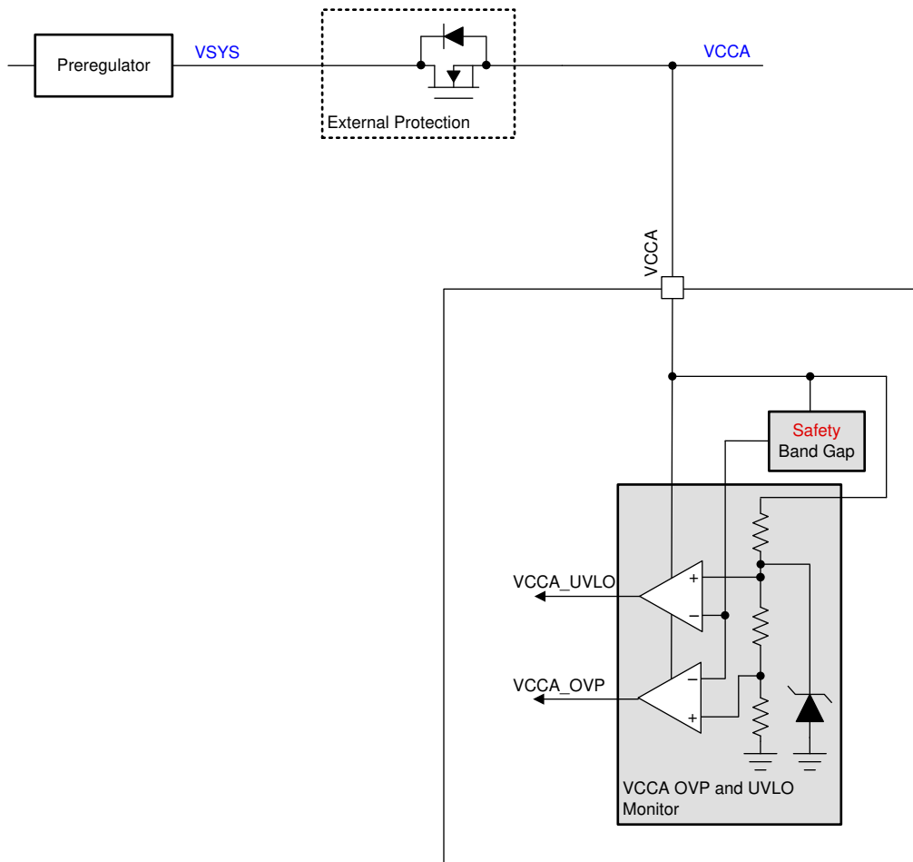
图 7-2. VCCA Monitor
