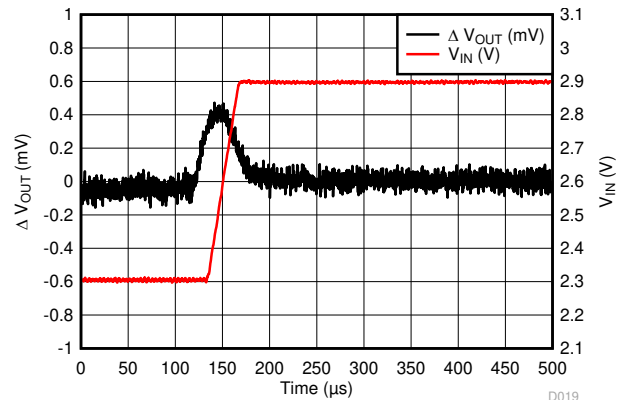
图 6-28. LP5912-1.8 Line Transient
