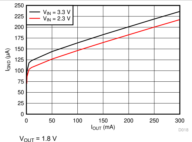
图 6-18. I_{GND} vs I_{OUT}
