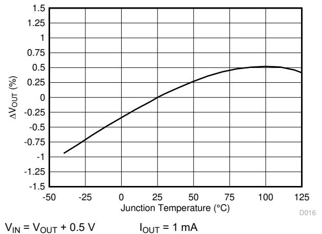
图 6-16. \Delta V_{OUT} vs Temperature
