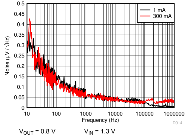
图 6-14. Noise Density
