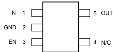
图 4-3. DBV 封装、5 引脚 SOT-23 (顶视图)
