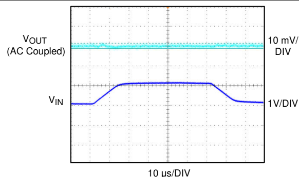
图 5-8. 线路调整
