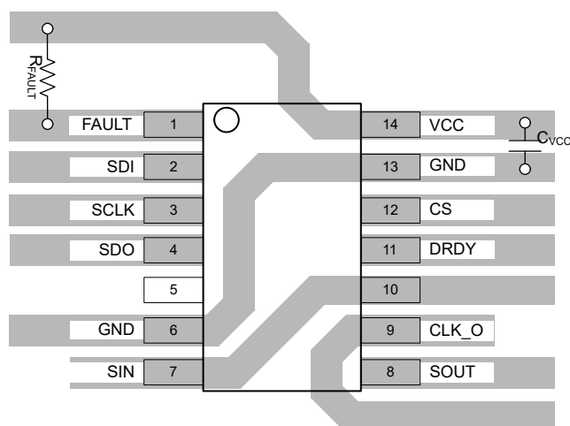
图 8-6. LP5899 布局示例
