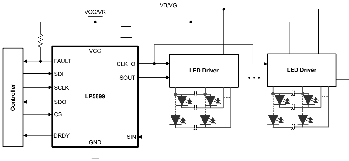
图 3-1. 典型应用图
