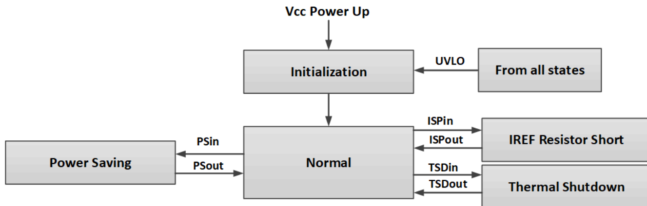
图 8-16. Functional Modes
