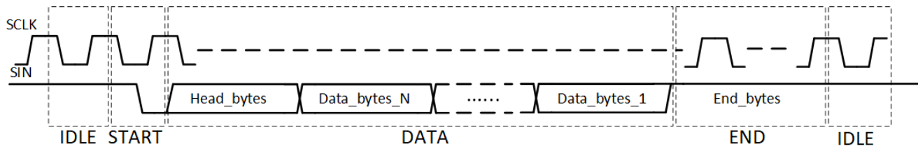
图 8-17. CCSI Frame
