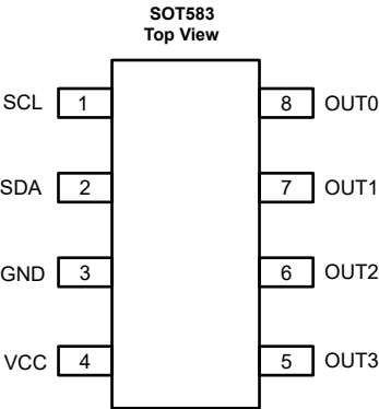
图 5-1. LP5816 DRL 封装 8 引脚 SOT583 顶视图
