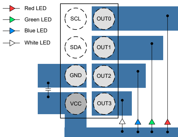
图 8-5. LP5816 YCH 封装布局示例
