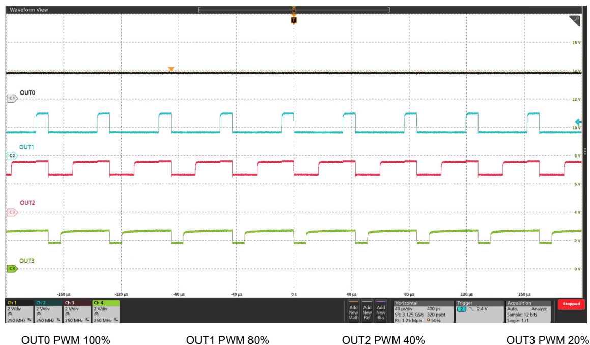
图 8-3. OUT0、OUT1、OUT2、OUT3 的电流阱波形
