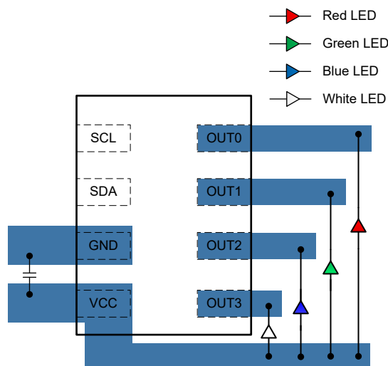
图 8-4. LP5816 DRL 封装布局示例
