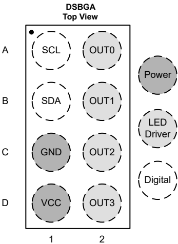
图 5-2. LP5816 YCH 封装 8 引脚 DSBGA 顶视图
