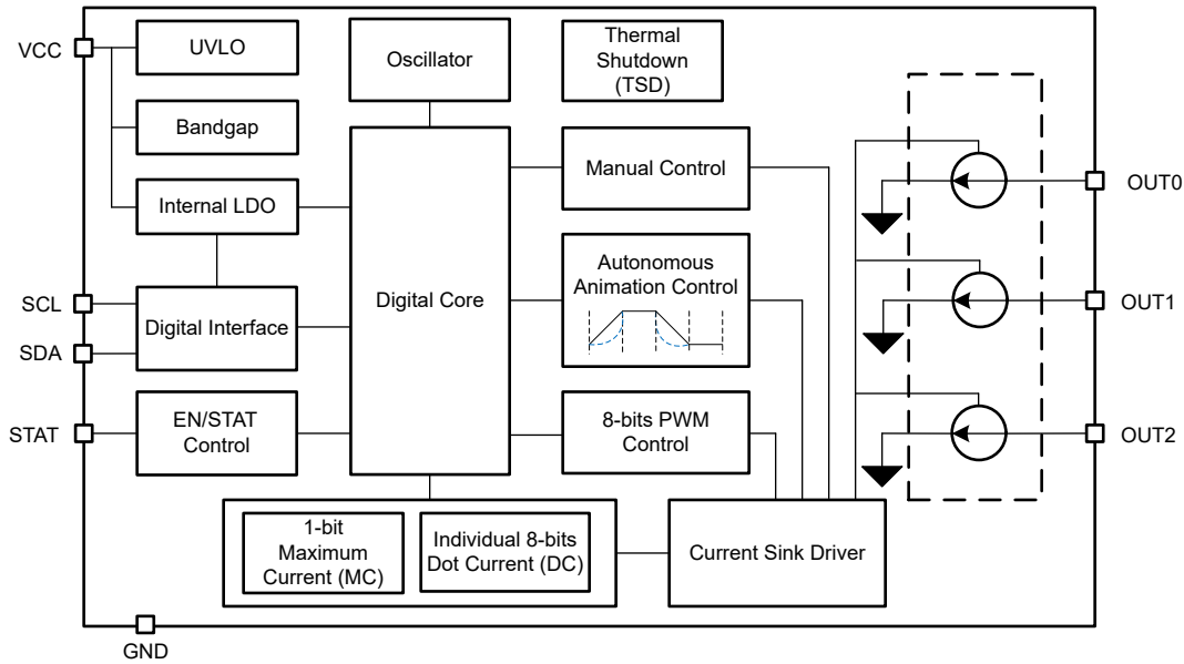
图 7-1. LP5815 功能模块
