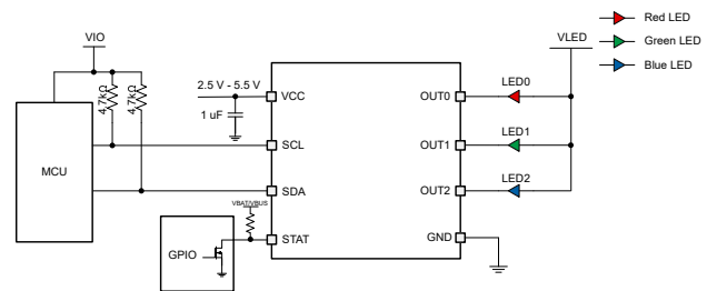
LP5815 简化原理图
