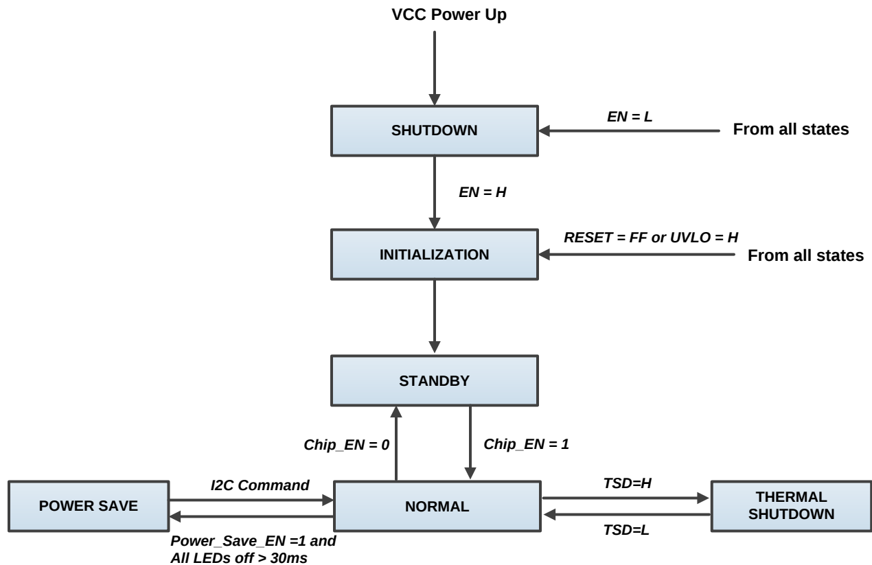
图 15. Functional Modes
