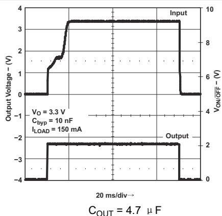
图 8-23. Turn-On Time
