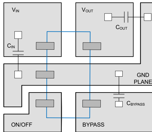
图 7-25. Layout Diagram
