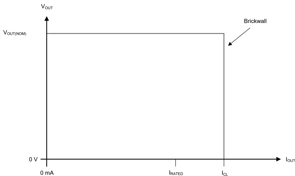
图 6-3. Current Limit
