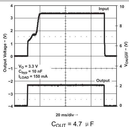
图 7-23. Turn-On Time
