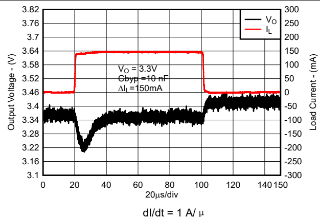
图 7-6. Load Transient for New Chip
