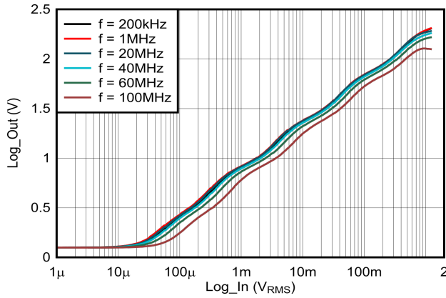
图 5-1. 各种频率下的输出
