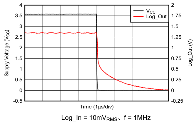
图 5-18. 电源斜降的关断时间
