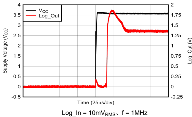
图 5-17. 电源斜升的启动时间
