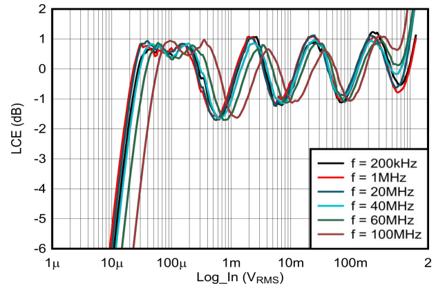
图 5-2. 不同频率下的对数相符性误差
