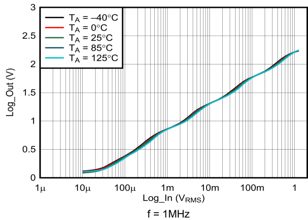
图 5-3. 各种温度点上的输出
