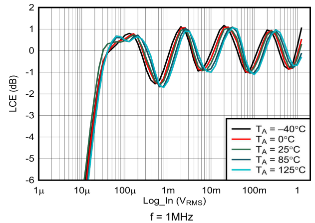
图 5-4. 不同温度点上的对数相符性误差
