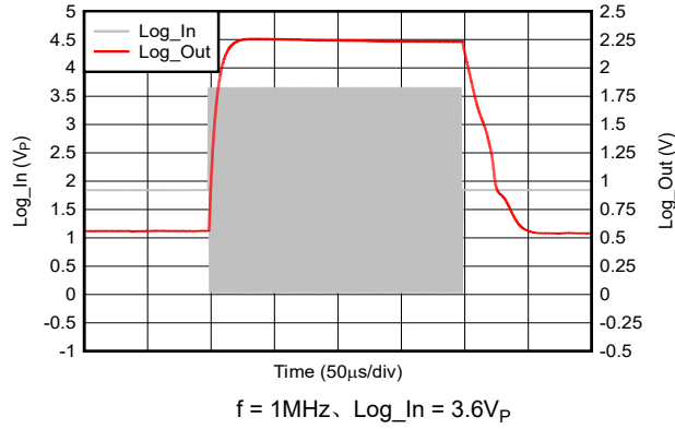
图 5-13. 过驱恢复
