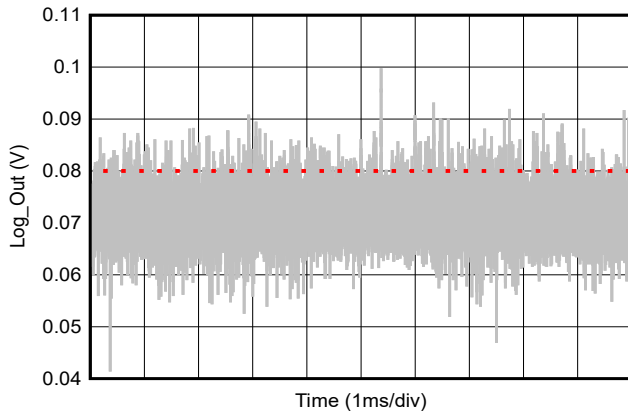
图 5-13. 过驱恢复
