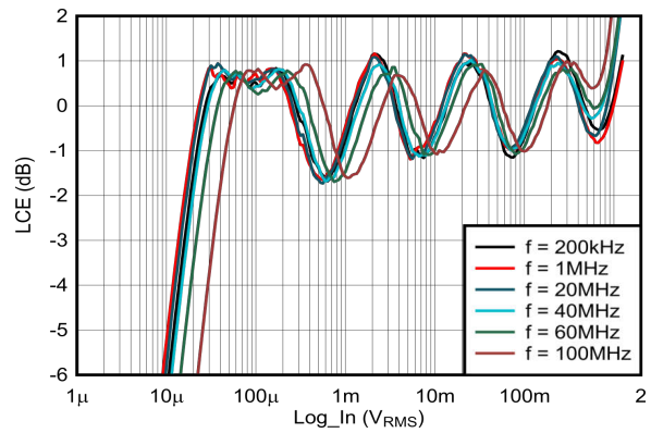
图 5-22. 不同频率下的对数相符性误差
