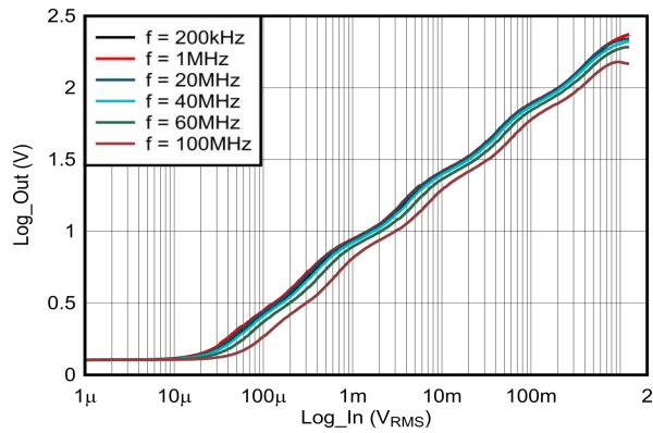
图 5-21. 各种频率下的输出
