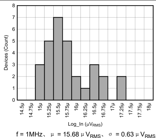
图 5-10. 最小 3dB 输入灵敏度
