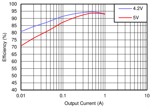
图 8-17. Efficiency
