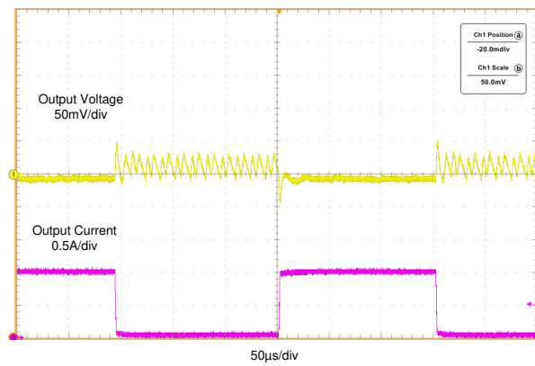
图 8-18. Load Transients In PWM Mode
