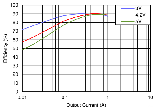
V_{OUT} = 1.8V 时自动模式下的典型效率
