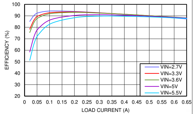
图 8-9. Efficiency V_{OUT} = 1.8\text{ V}
