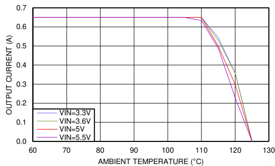
图 6-5. Thermal Derating V_{OUT} = 2.5\text{ V} , \theta_{JA} = 77^\circ\text{C/W}
