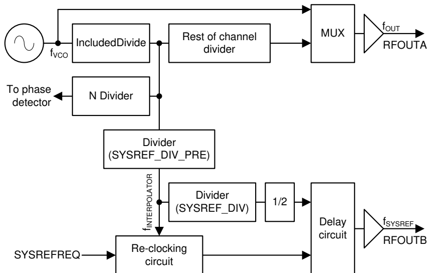
图 7-6. SYSREF Setup
