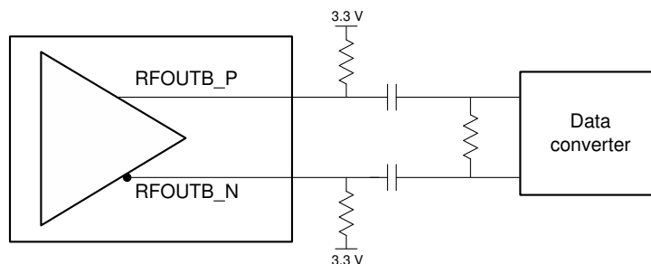
图 7-7. SYSREF Output
