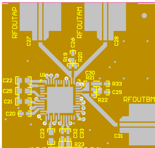
图 10-1. Layout Example
