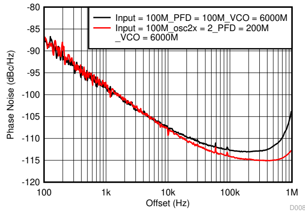
图 8-4. 100-MHz 输入 With OSCin Doubler
