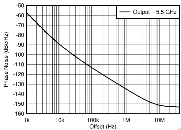
图 6-7. 5.5-GHz Output - Open-Loop Phase Noise
