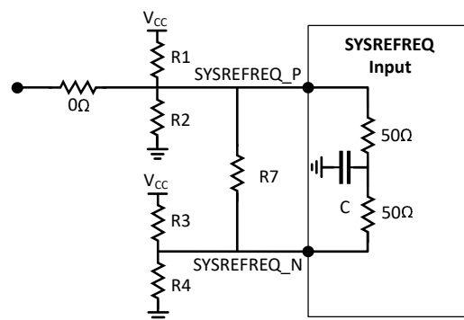
图 8-5. 直流耦合单端输入
