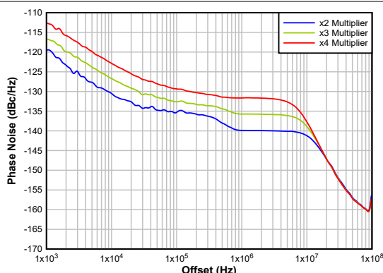
图 5-4. 6GHz 输出时的倍频器相位噪声图
