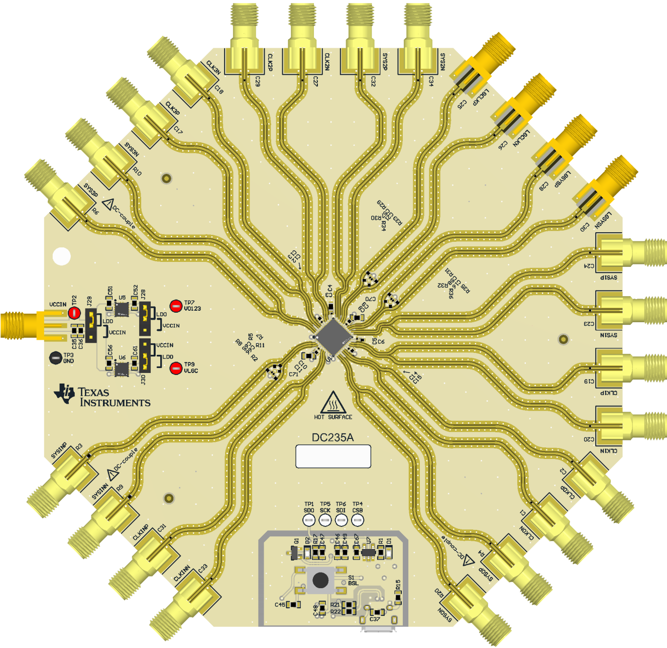
图 8-4. 布局示例
