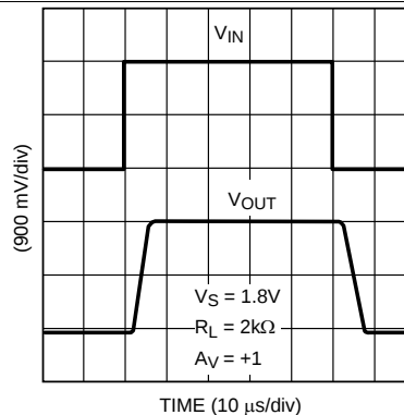
Figure 20. 大信号同相应
