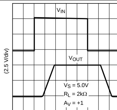
TIME (10 \mu s /div) Figure 26. 大信号同相响应
