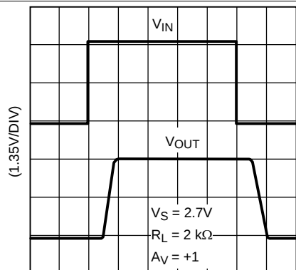
TIME (10 \mu s /DIV) Figure 25. 大信号同相响应
