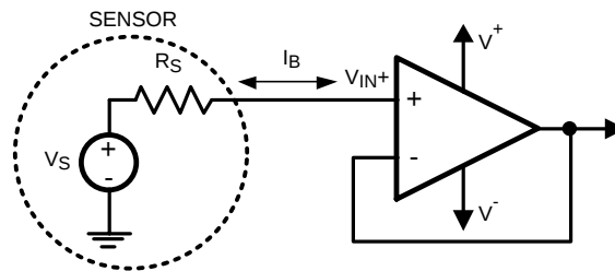
图 37. 高阻抗传感器接口
