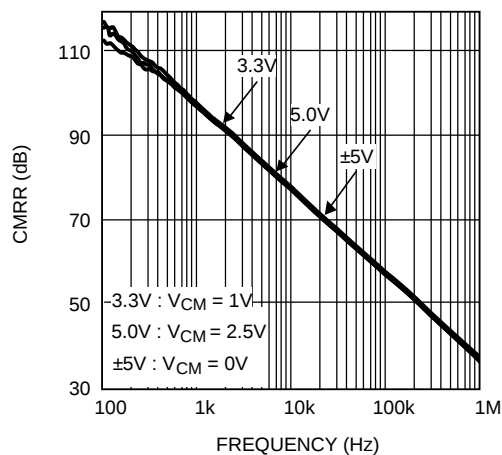
图 22. CMRR 与频率间的关系
