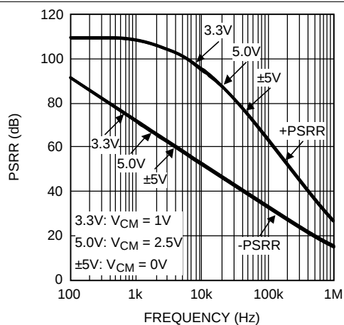
图 21. PSRR 与频率间的关系
