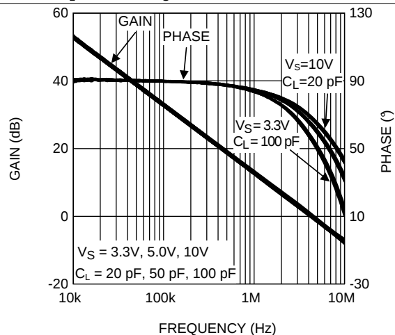
图 19. 不同负载条件下的开环频率响应
