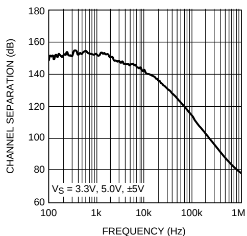
图 23. 通道分离与频率间的关系
