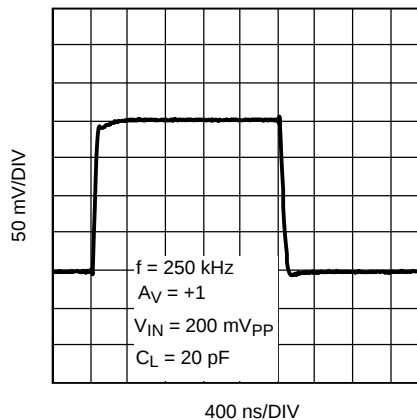
图 26. 增益 = 1 时的小信号阶跃响应
