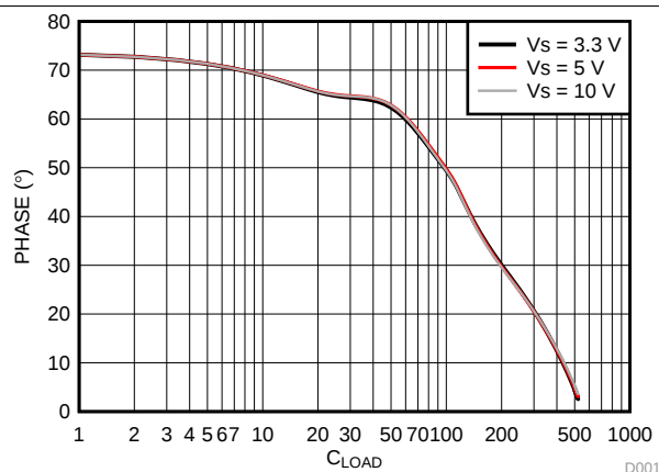
图 20. 相位裕度与 C_L 间的关系
