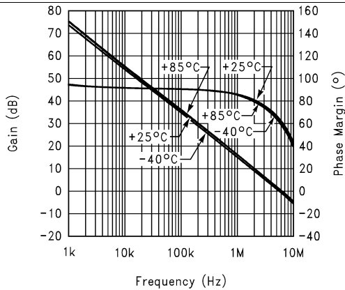
图 19. 增益和相位裕度与频率间的关系 ( R_L = 100k\Omega 、 2k\Omega 、 600\Omega ), 电压为 5V
