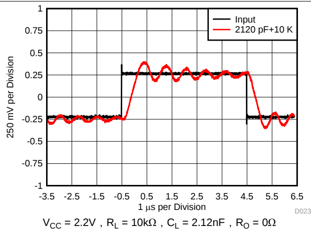
图 23. 脉冲响应
