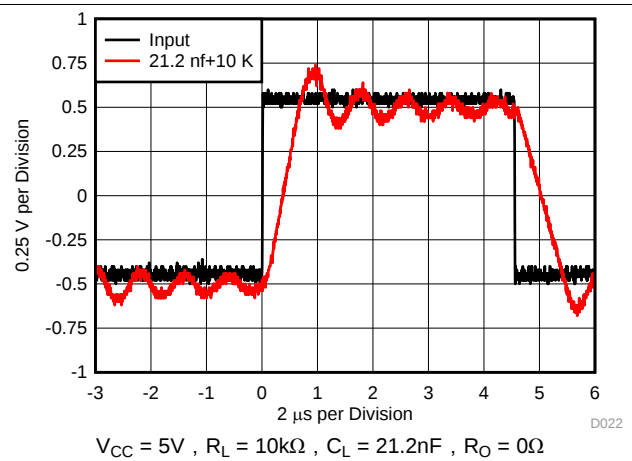
图 22. 脉冲响应
