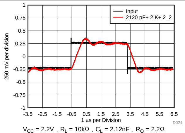
图 24. 脉冲响应
