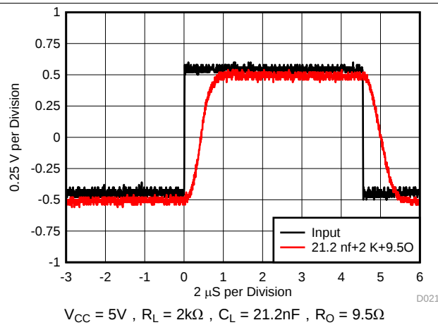
图 21. 脉冲响应
