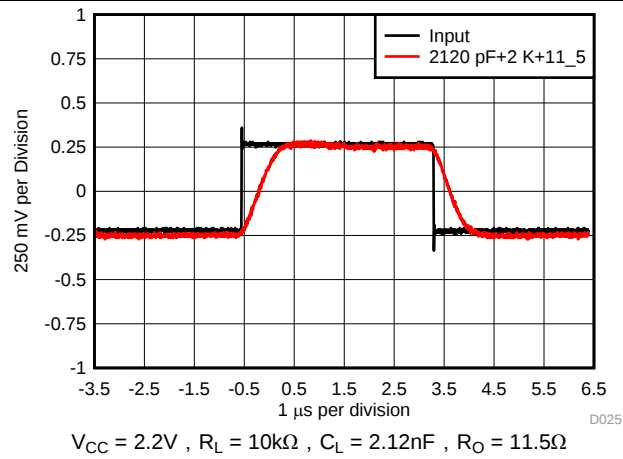
图 25. 脉冲响应
