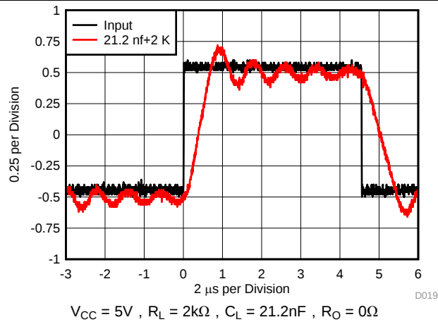
图 19. 脉冲响应
