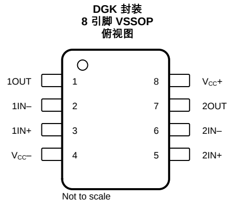
引脚功能
