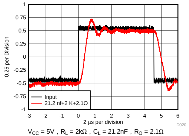
图 20. 脉冲响应
