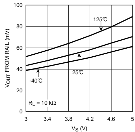
图 12. 正输出摆幅与电源电压间的关系
