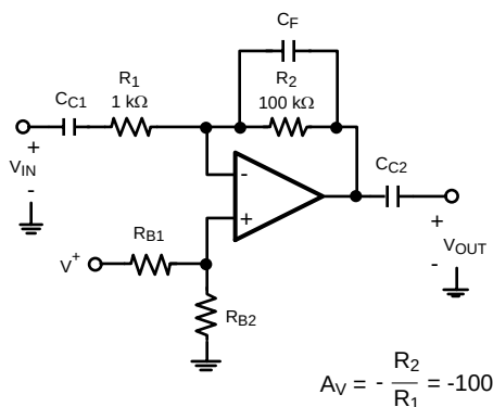
图 37. 高增益反相放大器
