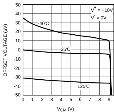
图 3. 失调电压与 V_{CM} 间的关系
