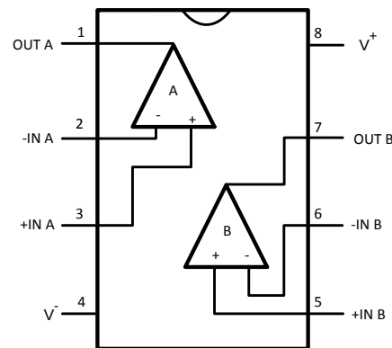
SOT-23 的 – LMV612
