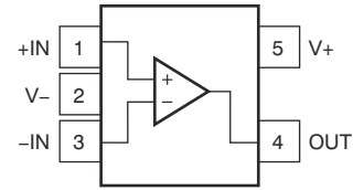
图 5-2. LMV321A-Q1 DCK, LMV321AU-Q1 DBV Package, 5-Pin SC70, SOT-23 (Top View)
