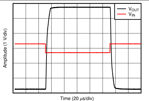
图 5-23. 过载恢复
