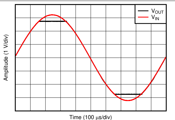
图 5-22. 无相位反转
